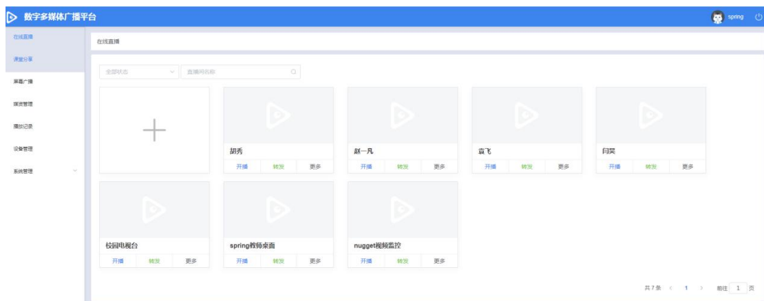
图 3-2-1 直播间列表
