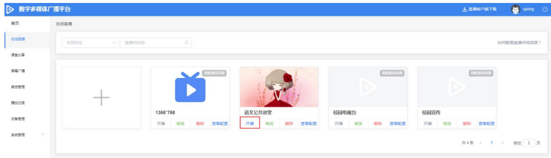
图 3-2-3-3 直播开播（一）
